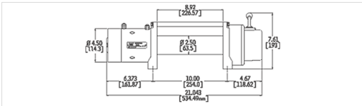
Winch Dimensions: 21.04" L. x 6.3" D. x 7.6" H. (534mm L. x 160mm D. x 193mm H.)
